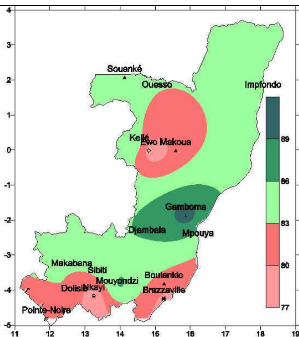
Fig5: Humidité moyenne de l'air sous abri de la 3e décade du mois de Mai 2019
