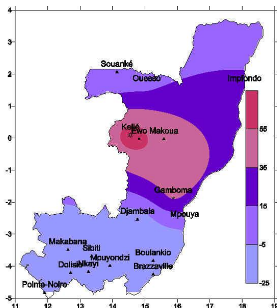
Fig3: Anomalies des précipitations de la 3e décade du mois de Mai 2019
