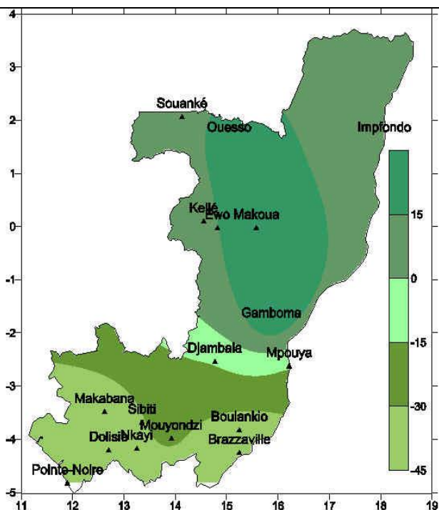
Fig4: Bilan hydrique de la 3e décade du mois de Mai 2019
