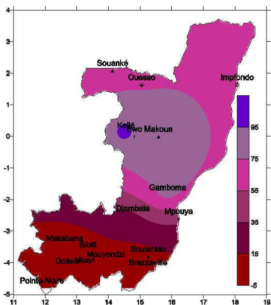
Fig2: Total des précipitations de la 3e décade du mois de Mai 2019
