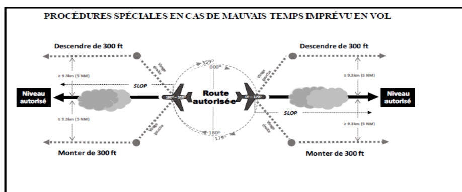
Figure 15-2. Guide visuel sur les procédures de déroutement en cas de mauvais temps si une autorisation ATC révisée ne peut pas être obtenue (voir section 15.2.4.3)
