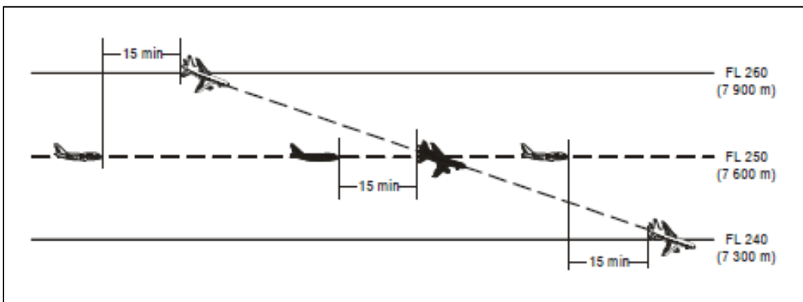
Figure 5-19B. Séparation de 15 minutes entre aéronefs en descente sur des routes convergentes [voir § 5.4.2.2.2.2, alinéa a)]
