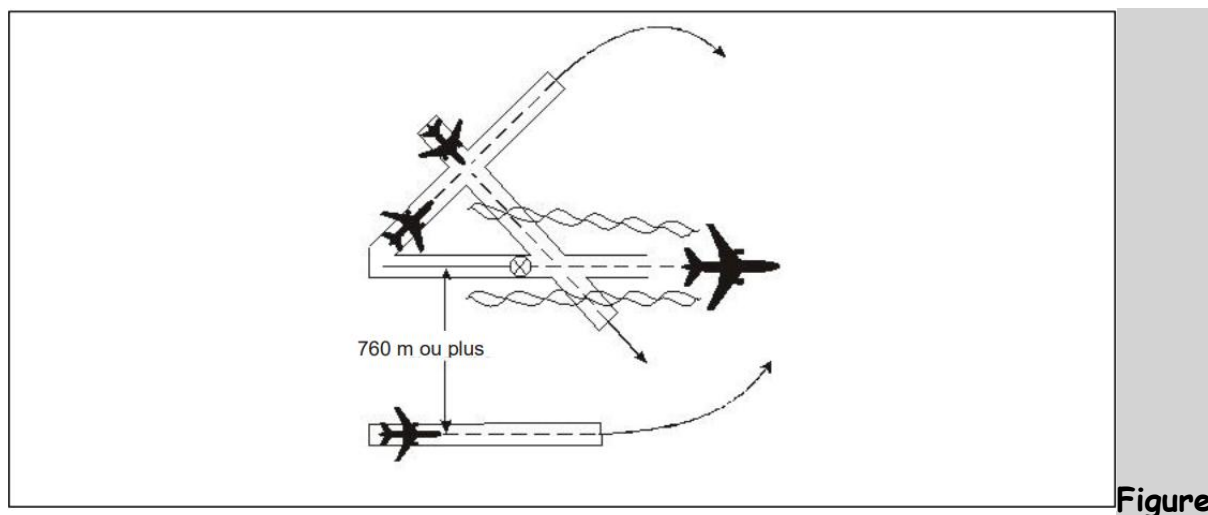
Figure 5.43. Séparation en fonction de la turbulence de sillage, pour l'aéronef qui traverse le sillage [voir § 5.8.3.1, alinéas c) et d) et § 5.8.3.2, alinéas c) et d)]
