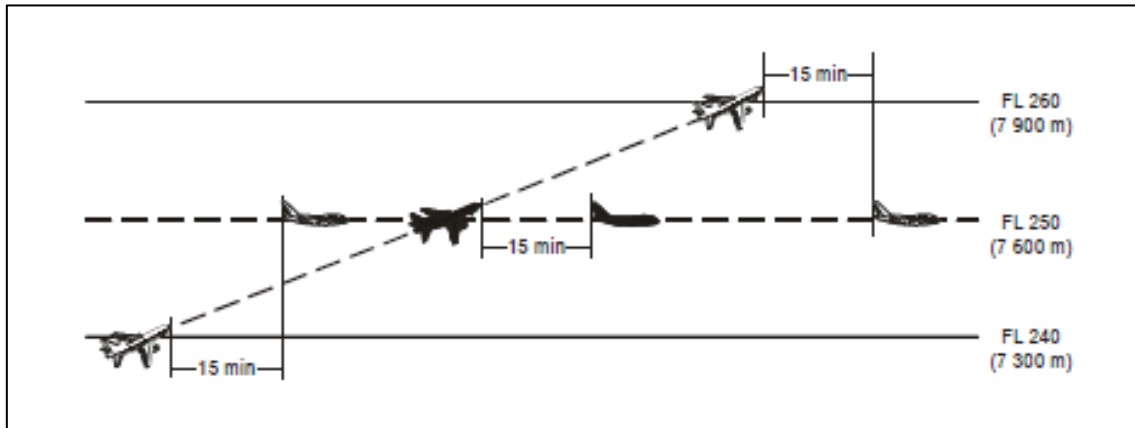
Figure 5-19A. Séparation de 15 minutes entre aéronefs en montée sur des routes convergentes [voir § 5.4.2.2.2.2, alinéa a)]
