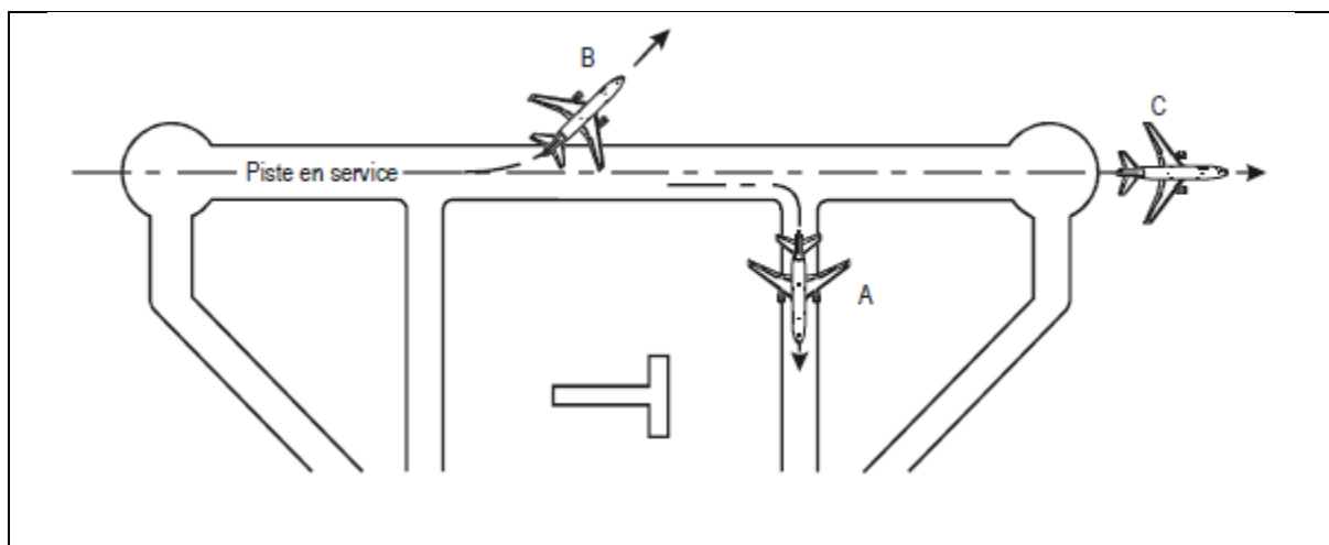
Figure 7-2. Séparation entre les aéronefs à l'arrivée et au départ (voir Sections 7.9.2 et 7.10.1)
