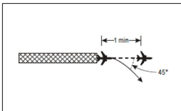
Figure 5-37. Séparation d'une minute entre aéronefs au départ qui suivent des routes divergeant d'au moins 45 degrés (voir § 5.6.1)
