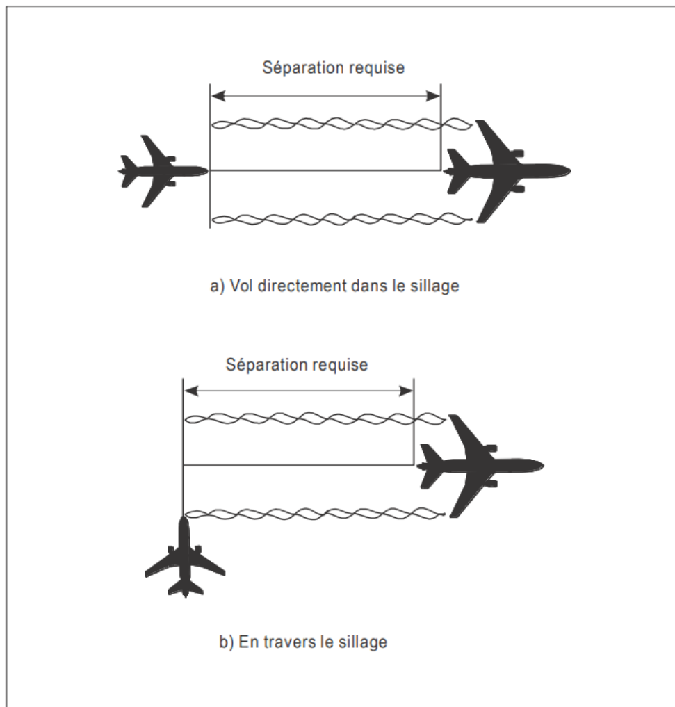
Figure 8-1 : Vol directement dans le sillage et en travers du sillage (voir § 8.7.3.4 et 8.7.3.5)
